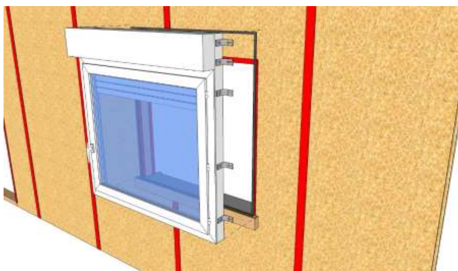
Figure 34 – Présentation de la menuiserie pré-équipée des équerres de fixation
