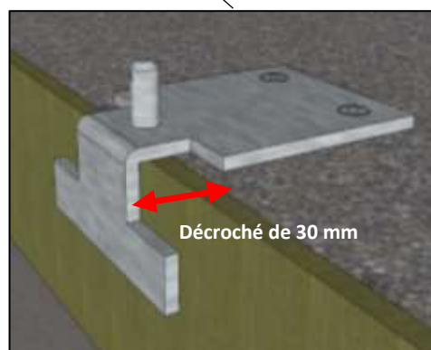
Figure 20 – Pose des platines support du système d'ancrage LogiFix®Rideau en bord de dalle (réglage de l'aplomb de la façade) et mise en œuvre de la laine de roche en nez de dalle et de refend (cas des façades indépendantes par niveau)
