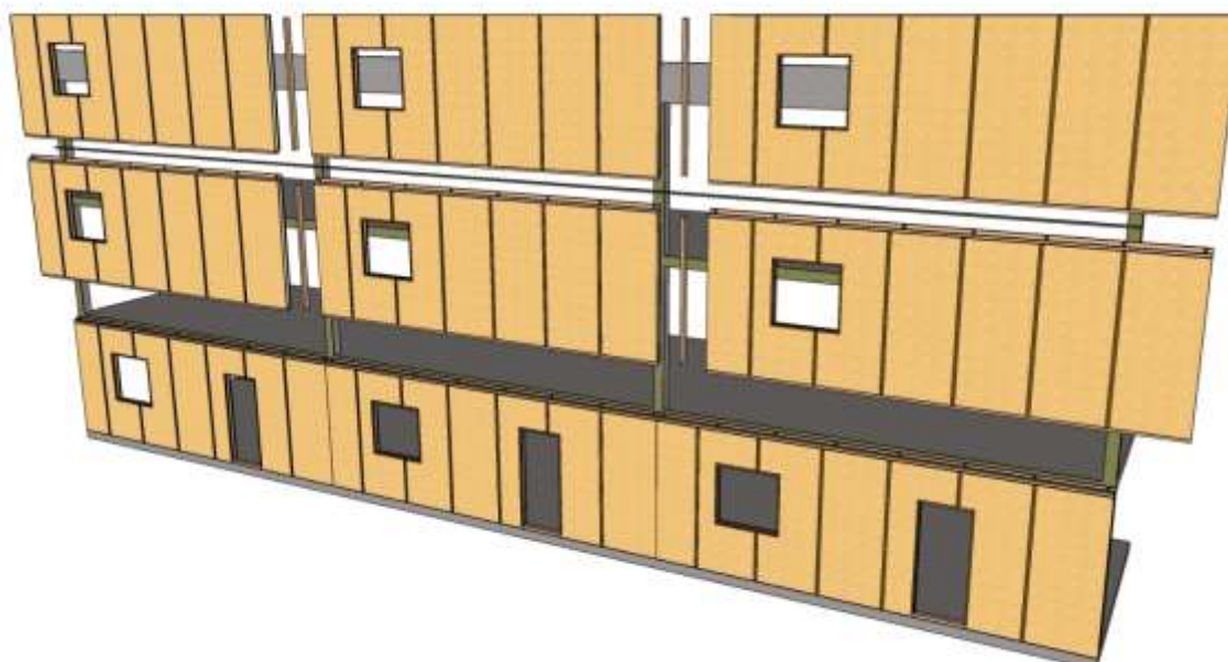
Figure 16 – Pose de l'ensemble des panneaux (cas des façades autoportantes)
