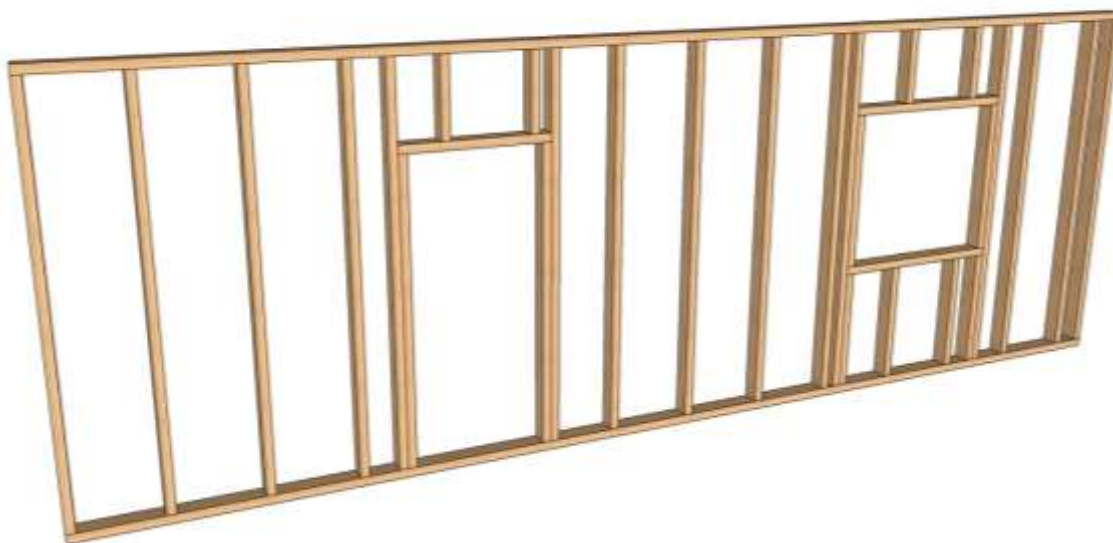
Figure 5 – Vue de l'ossature bois intérieure d'un panneau de façade LogiSkin
