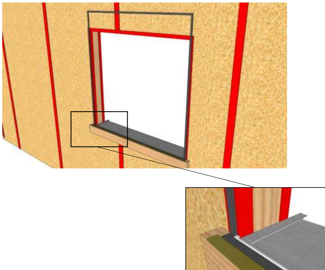
Figure 33 – Pose d'une cale en bois dur sur la traverse bois d'appui de menuiserie et pose d'un joint en mousse imprégnées précomprimées en périphérie de l'ouverture
