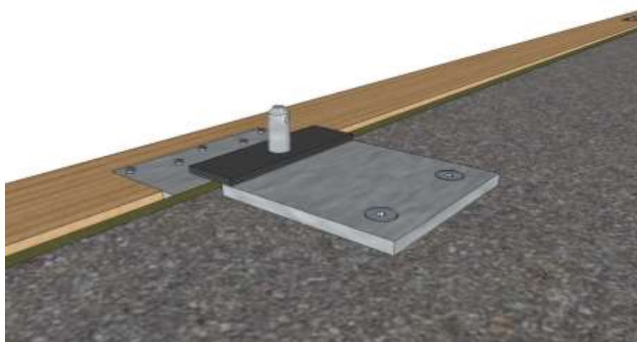
Figure 25 – Mise en place de cales pour régler le niveau général de la dalle (cas des façades indépendantes par niveau)
