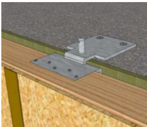
Figure 24 – Bride fixée, autorisant un déplacement vertical de la dalle +/- 15 mm (cas des façades indépendantes par niveau)
